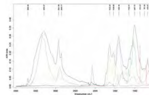
ФИГ. 4. ИЧ-ФТ спектър при отслабено пълно вътрешно отражение (ATR) на проба K1 (в черно) и референтни материали пруска синя (в синьо), калциев карбонат (в червено), яйце (в оранжево) и целулозна нишка (в зелено)
