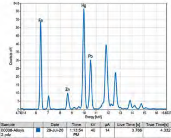
ФИГ. 17. XRF спектри на кафява цвeтна партия. S1 Titan Bruker
