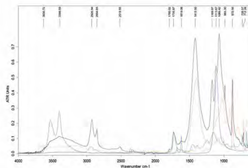
ФИГ. 8. ИЧ спектър при отслабено пълно вътрешно отражение (ATR) на долната страна на проба К3 – жълто (в черно) и референтни материали: калциев карбонат (в розово), гипс (в синьо), жълта охра (в оранжево) и полимеризирало масло (в зелено)
