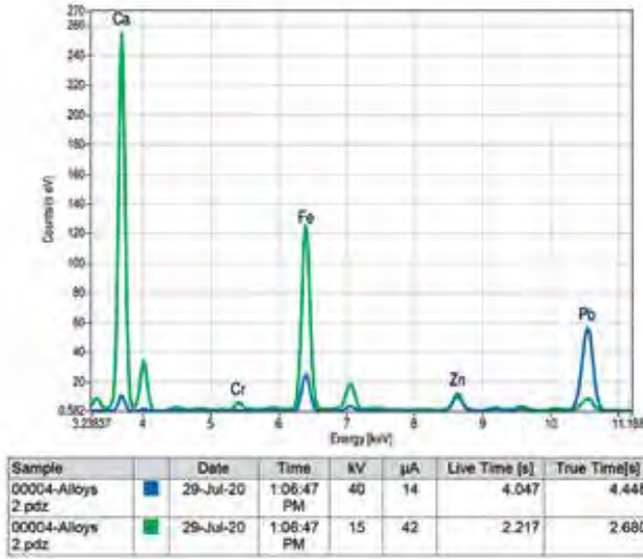
ФИГ. 16. XRF спектри на червени пигменти. S1 Titan Bruker а. Зона 6; б. Зона 7; в. Зона 8
