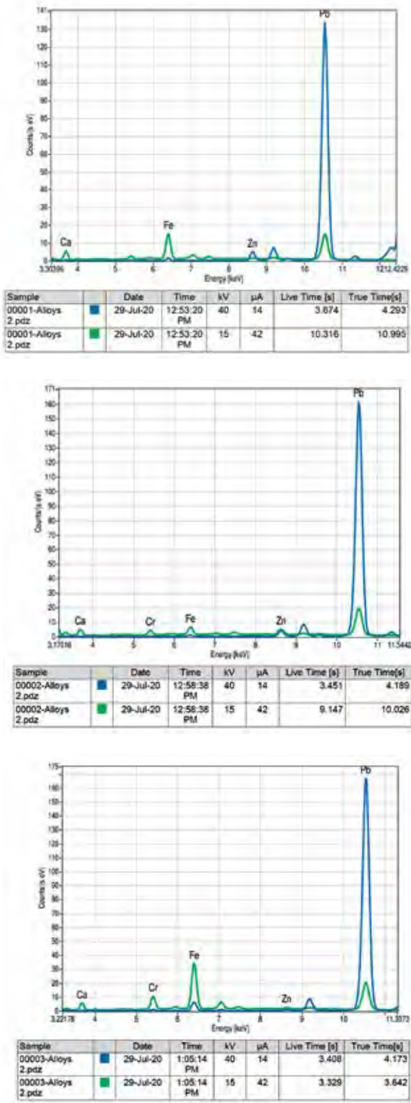
ФИГ. 12. XRF спектри на жълти пигменти. SI Titan Bruker а. Зона 1; б. Зона 2; в. Зона 3
