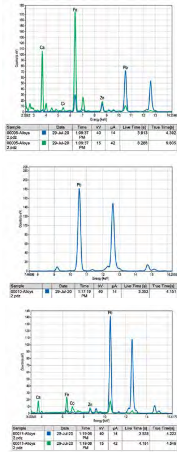
Горе: ФИГ. 13. XRF спектри на сини партии. S1 Titan Bruker А. Зона 5; Б. Зона 10; В. Зона 11 На с. 51, долу: ФИГ. 15. XRF спектри на грунда. S1 Titan Bruker А. Зона 13; Б. Зона 14
